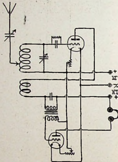
Fig. 4. De kortegolfontvanger.
